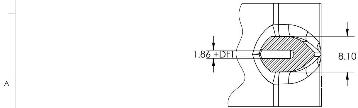
SECTION B-B SCALE 2 : 1
